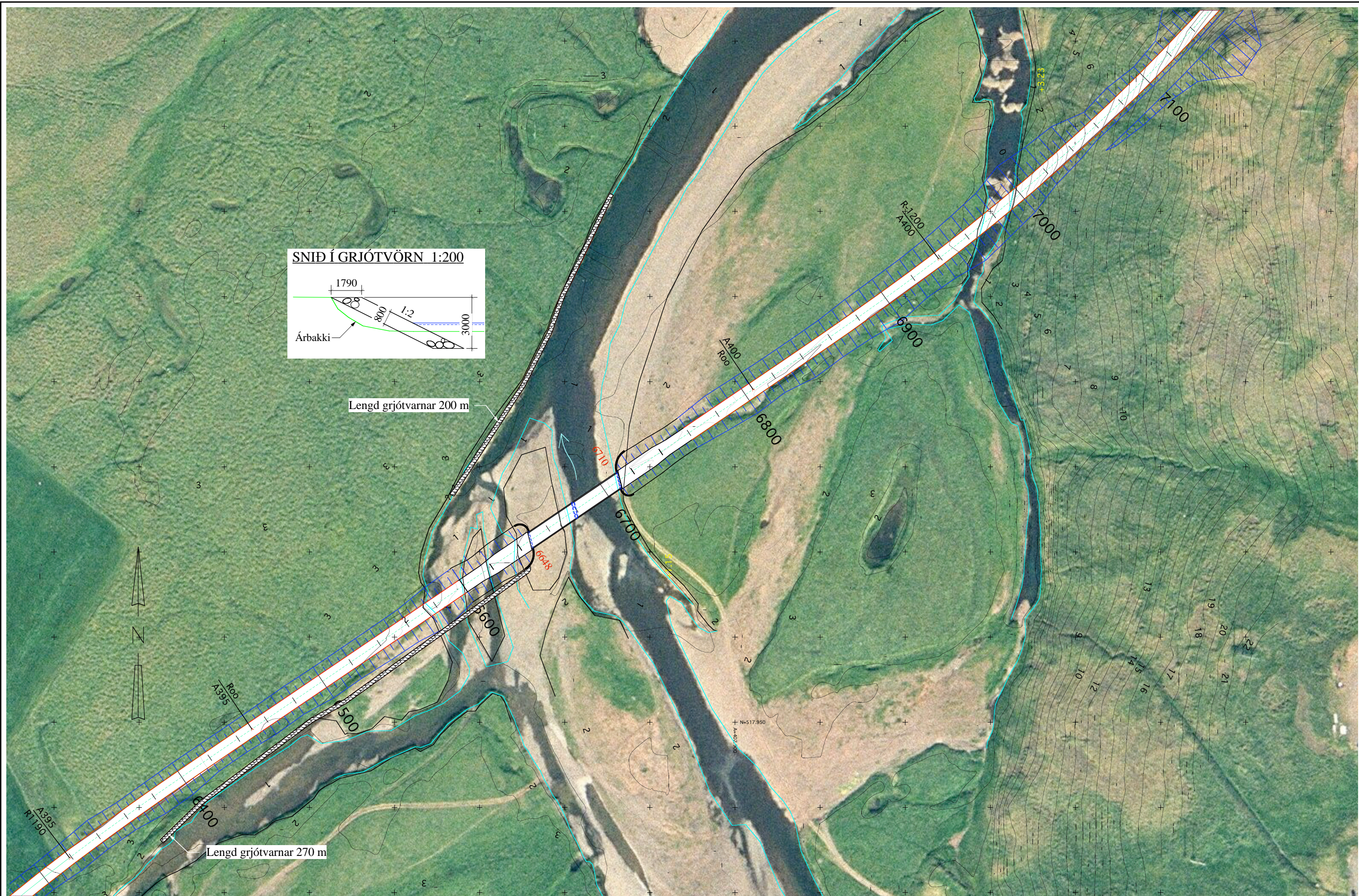
AFSTÖÐUMYND 1:2000
