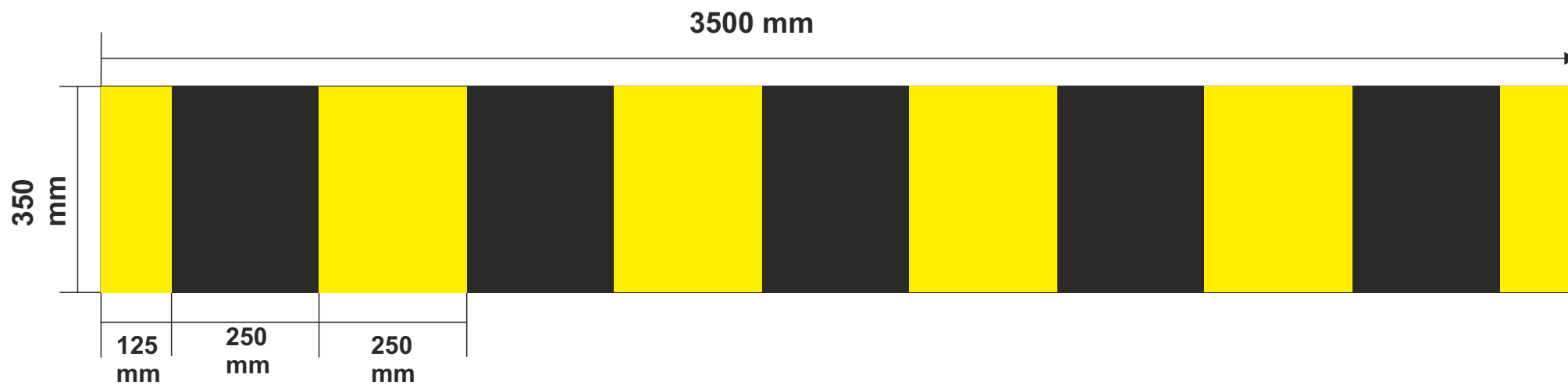
K21.11 Þverslá vegna hæðartakmarkana
